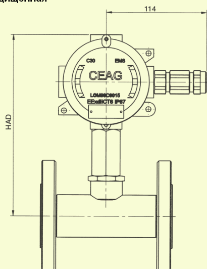
Взрывозащищенная оболочка
